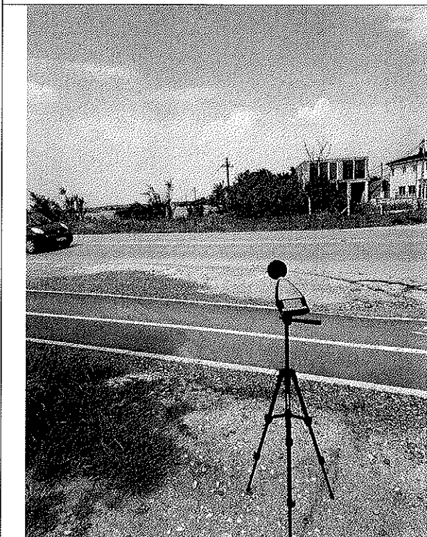
Slika 7 Merno mesto 3
